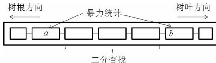
图12-34 实现 \text{update}(a, b, v, \text{res1}, \text{res2})
