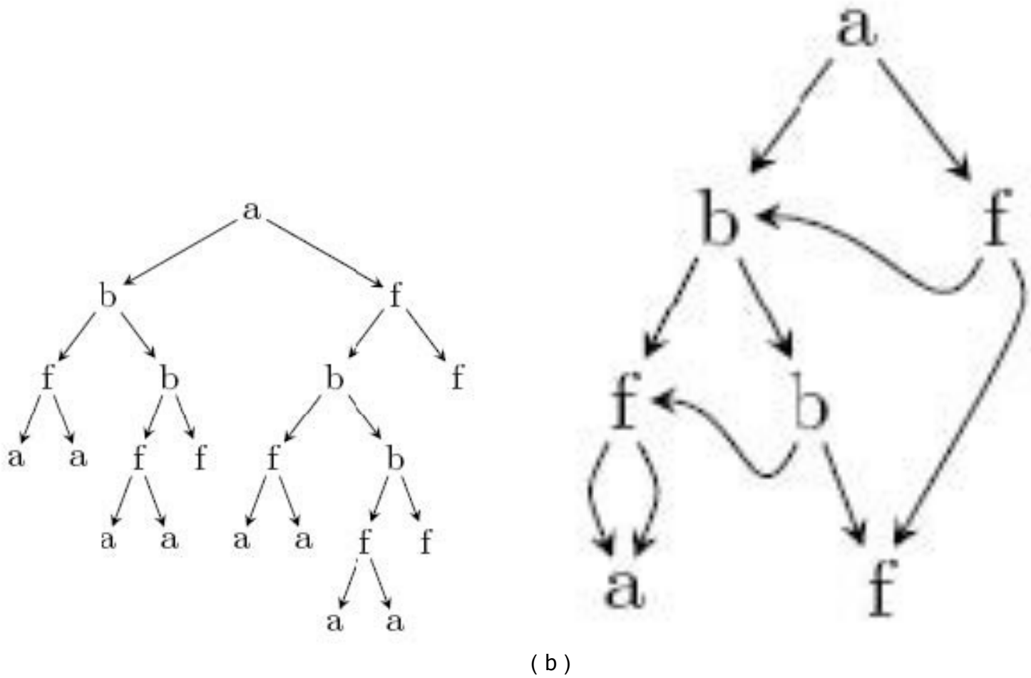
图11-3 公共表达式消除
