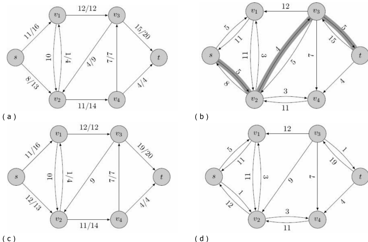
图11-10 残量网络和增广路算法
