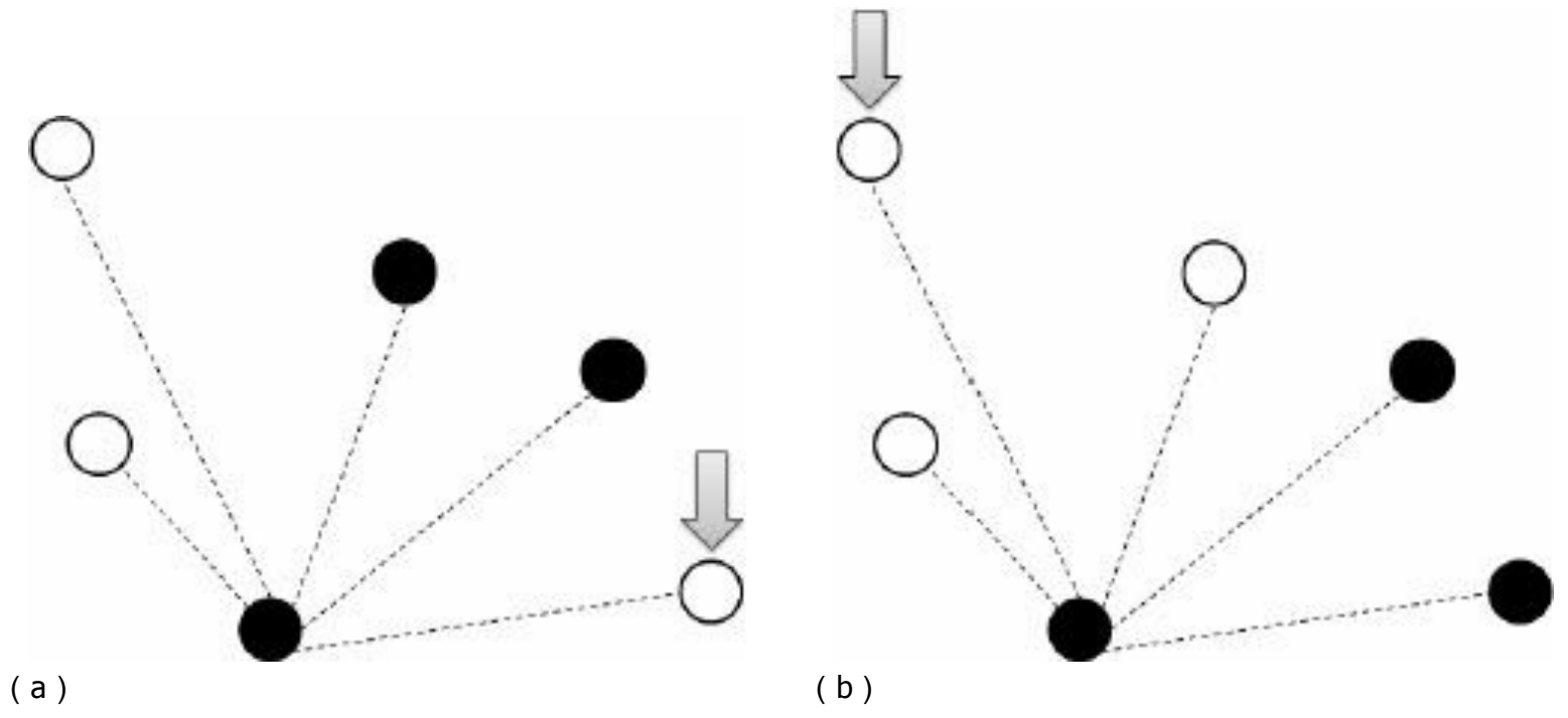
图8-6 巨人与鬼问题
