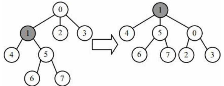
图11-1 无根树转有根树
