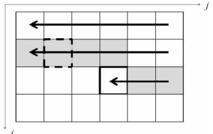
图9-6 0-1背包问题的计算顺序
