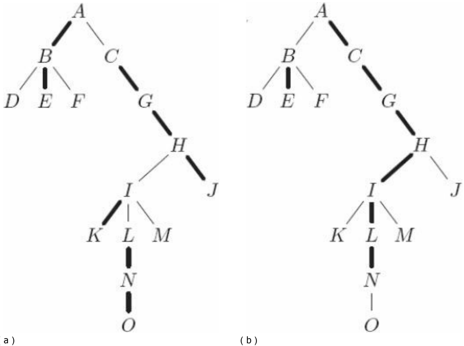
图12-13 Link-Cut树中Access操作
